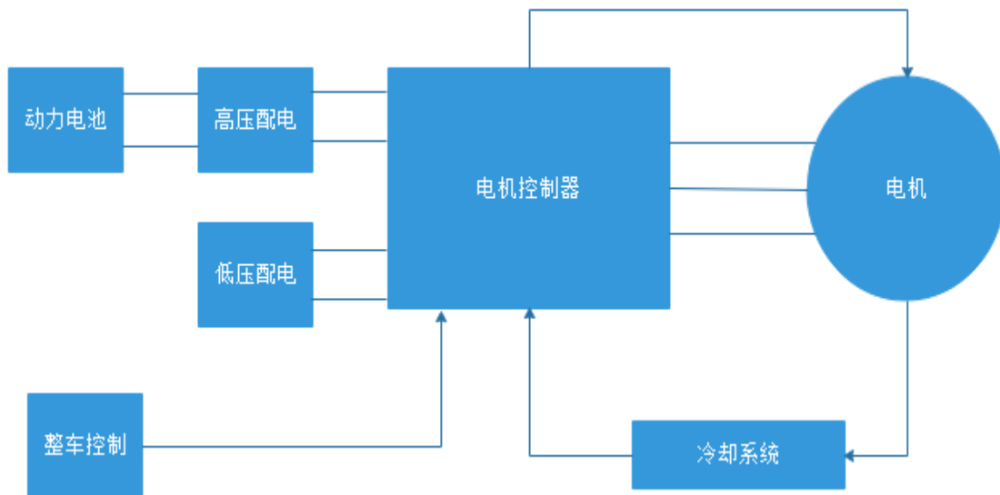
图5-1 电气连接示意图
