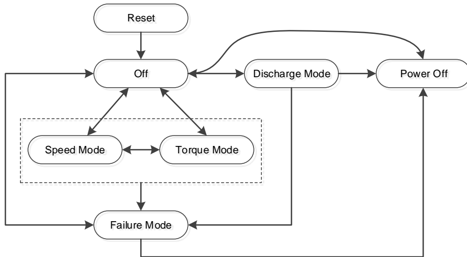
图4-1 MCU 工作模式转换关系图
