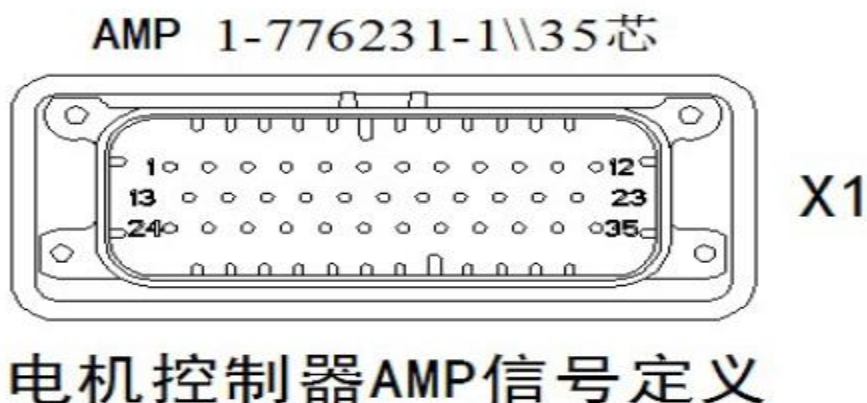
图5-2 电控低压插件
