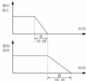
图5-9-5 V/F分离频率/电压先后下降示意图
