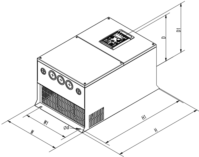
图 A1-2 外形示意图
