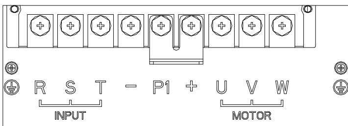
图 2-5 3PH 380V 37-160kW 主回路端子接线
