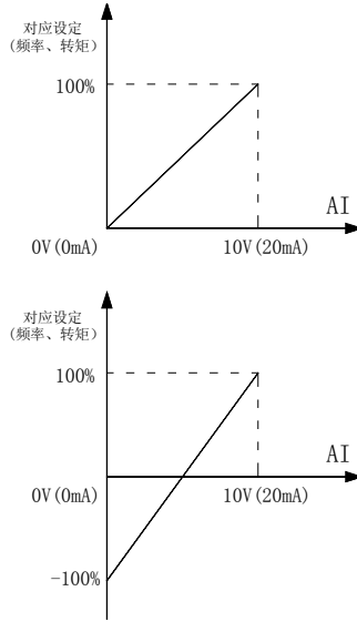
图5-2-5 模拟给定与设定量的对应关系
