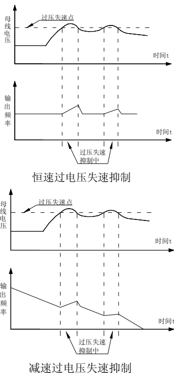
图5-9-8 过压失速动作示意图
