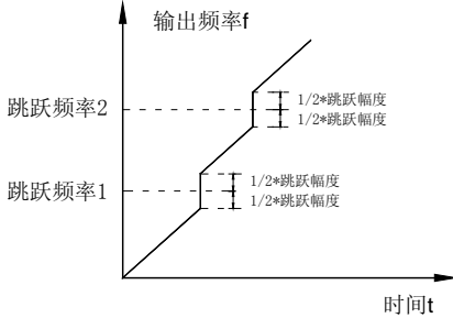
图5-5-5 加减速过程中跳跃频率有效示意图
