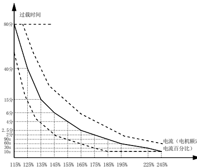
图5-B-1 电机过载保护反时限曲线示意图
