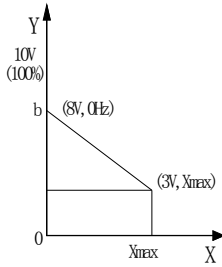
图5-3-2 带零偏或增益时的输出示意图(电压型)
