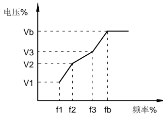
图5-9-2 多点V/F 曲线设定示意图
