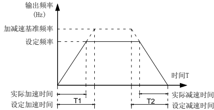
图 5-0-2 加减速时间示意图
