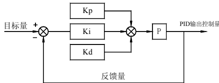
图5-6-1 过程PID 原理框图
